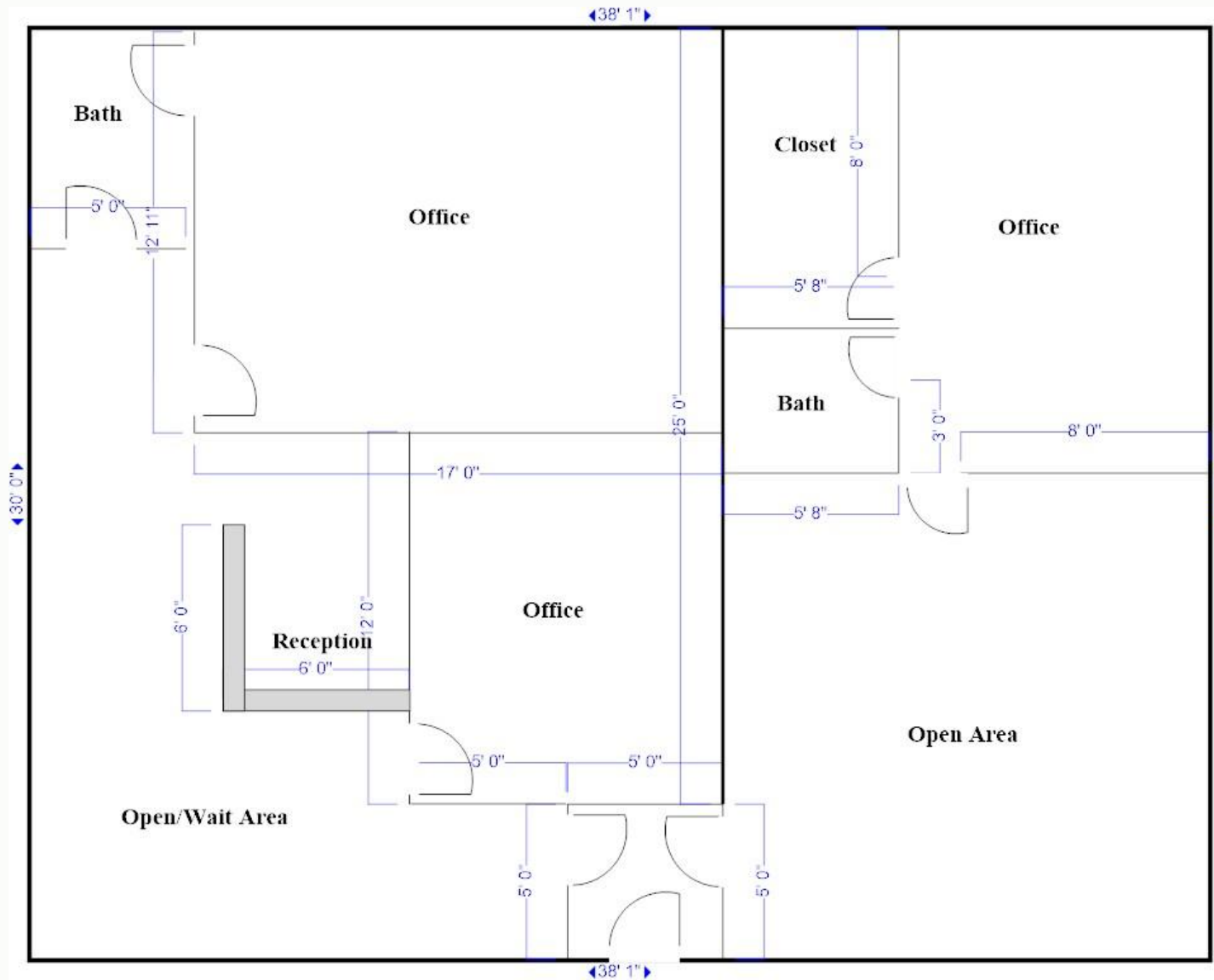
FloorPlan D24
